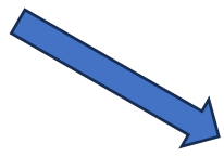
Mitgliederportal
