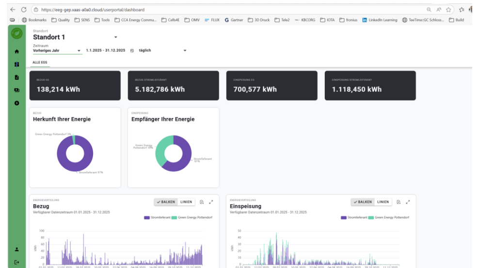
Mitgliederportal
