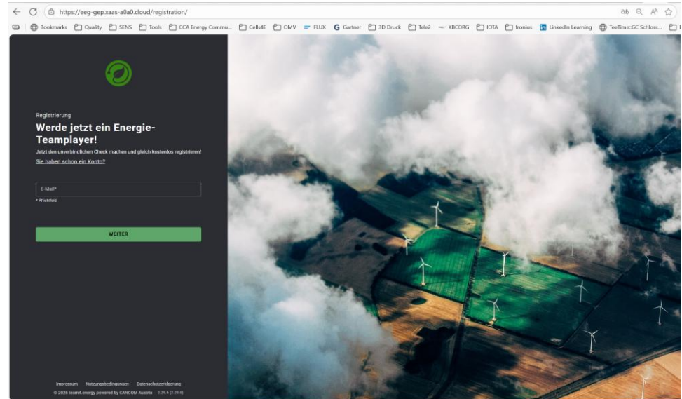
Mitglieder-Registrierung
