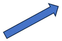
Mitglieder-Registrierung
